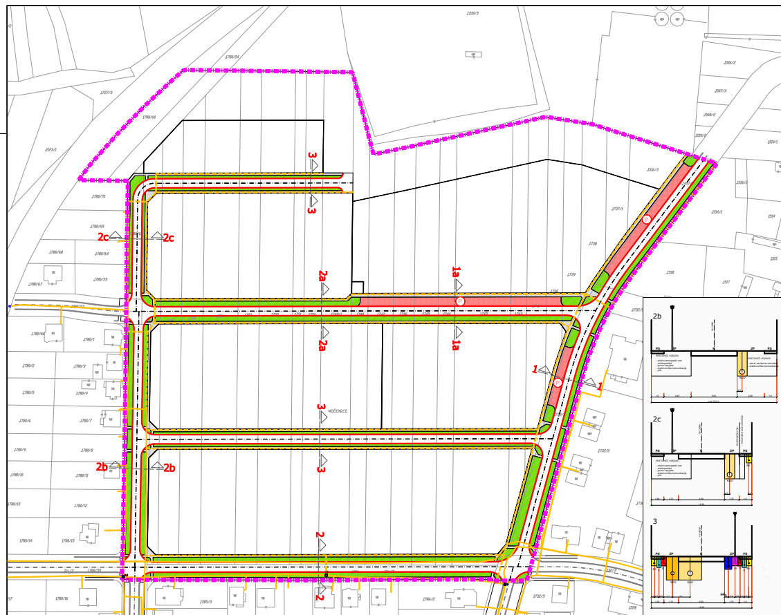
KARAKTERISTIČNI POPREČNI PRESJECI CESTA-ULICA MJ 1:200
