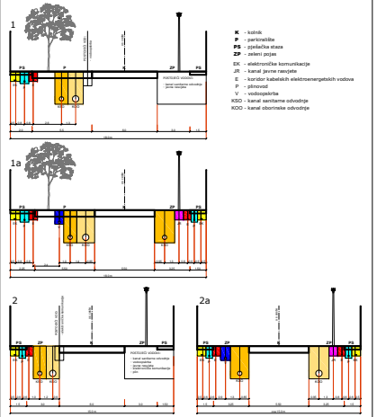
KARAKTERISTIČNI POPREČNI PRESJECI CESTA-ULICA MJ 1:200
